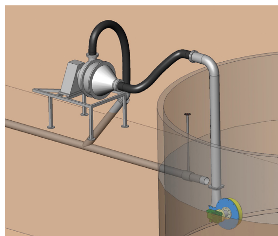
Eksempel på opstilling med Doda pumpe og turbofiller.
